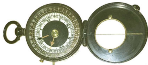
Marschkompass Urmodell von Francis Barker
