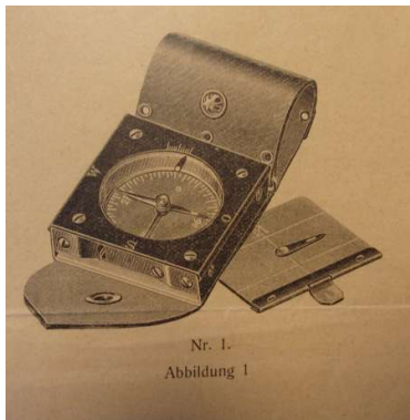
Modell Nr. 1 „Orion“
