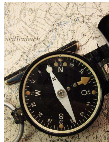
Ermitteln der Marschrichtung aus der Karte
