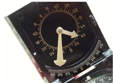
Inklinometer und Marschrichtungsanzeiger
